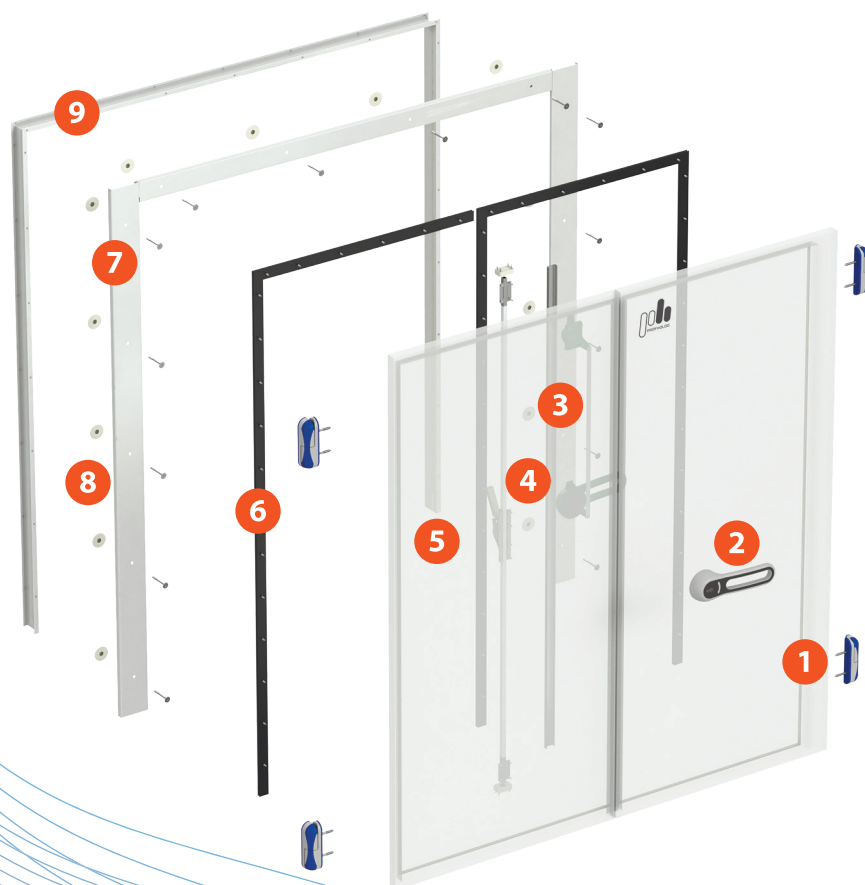
Рисунок 1. Распашная двустворчатая дверь
